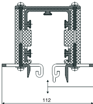
A-A geöffnet
