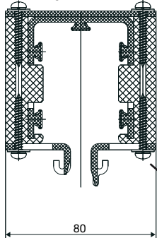
A-A geschlossen
